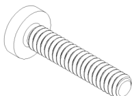
2x Vite M4x20 con intaglio a croce
