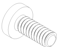
2x M4x14 Vis à empreinte cruciforme ( SP4 )
